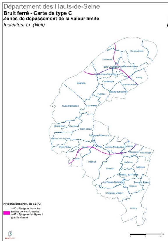
Figure 8 : carte de type C – Indicateur Ln
